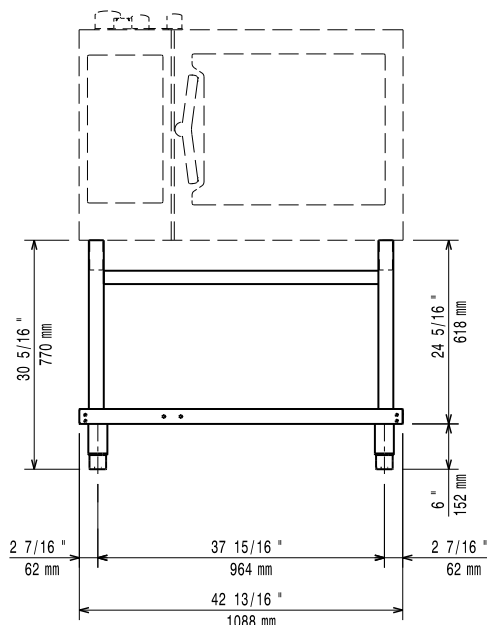
Zij aanzicht
