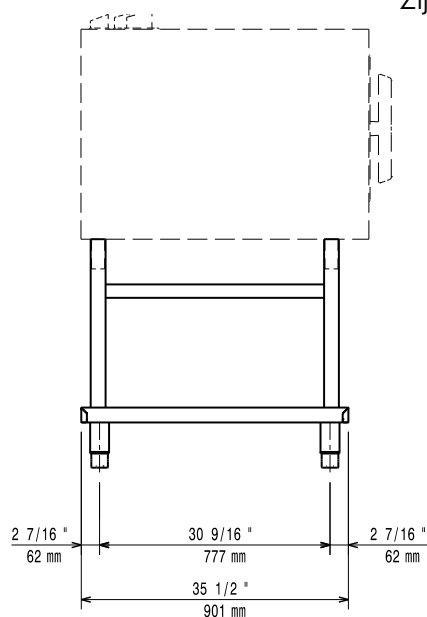
Boven aanzicht
